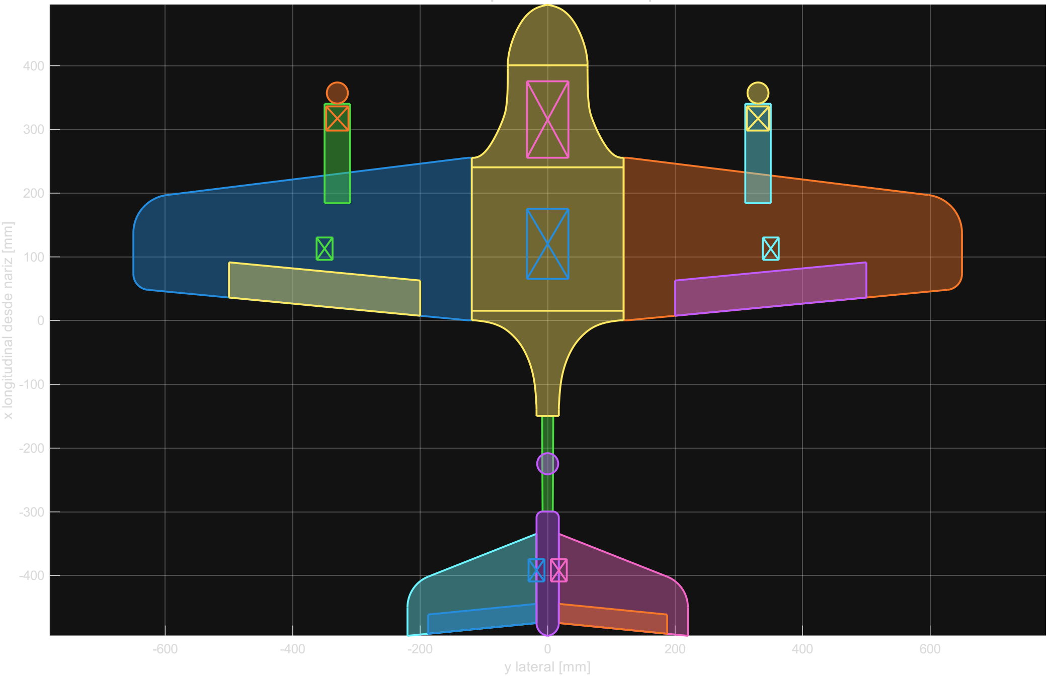
Partes DXF separadas con area transparente
